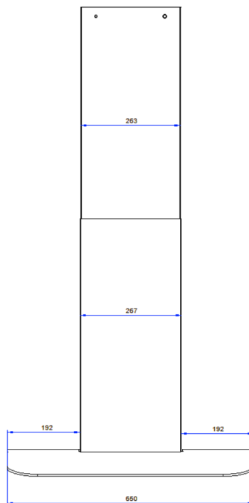
Sivulta
